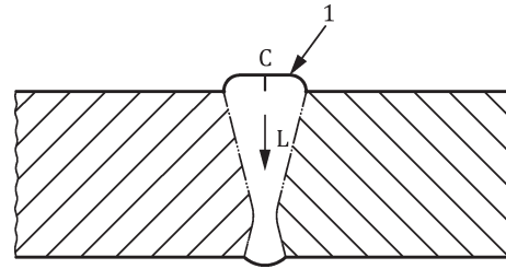
b) Longitudinal waves, L
