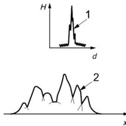
a) probe position of A-scan and variation in signal amplitude (widok A-skanu i rozrzut w wysokości wzmożenia sygnału)
