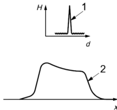
a) probe position of A-scan and variation in signal amplitude (widok A-skana i zróżnicowanie w przebiegu wysokości echa)
