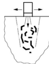
c) ultrasonic response in lateral (length) direction (typowy widok przy przesuwie bocznym wzdłuż spoiny)
