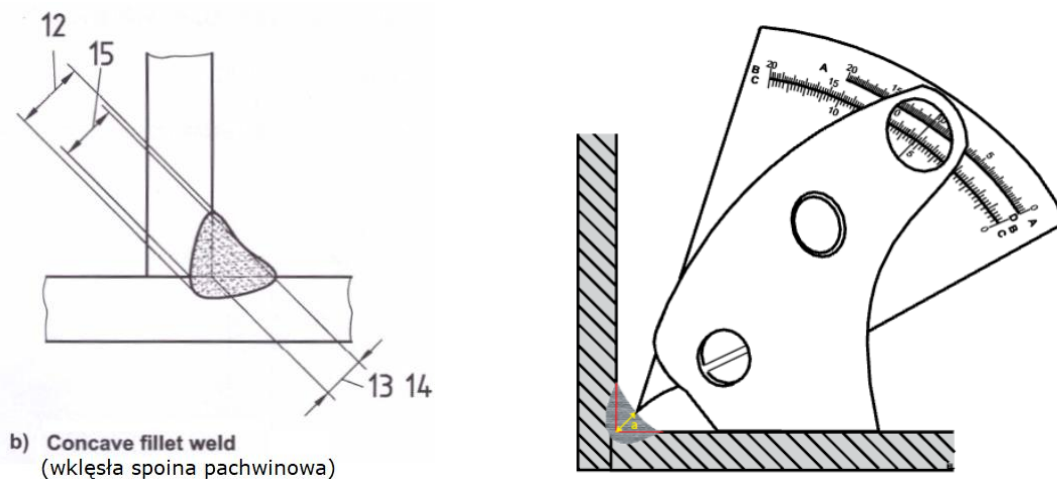
Rysunek 5. Bezpośredni pomiar wartości a w przypadku spoiny wklęsłej lub płaskiej 12) najwyższa wysokość pachwiny, 13) projektowa grubość pachwiny, 14) rzeczywista grubość pachwiny, 15) efektywna grubość pachwiny
