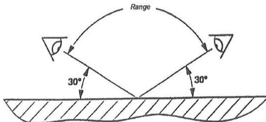
Rysunek 1. Prawidłowy dostęp do wykonania badania Figure 1. Proper access for testing conduction
